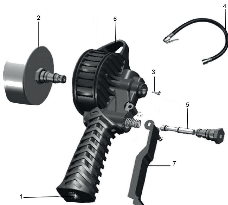
Bild 1. Baugruppen
